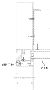
〈참고도면 1〉 설치 상태
