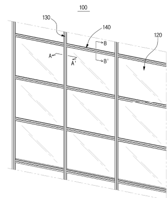
〈도 1〉 커튼월 창호 설치상태도
